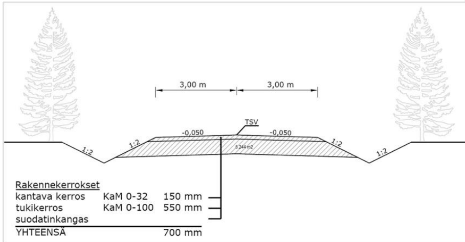
Kuva 3-3. Periaatekuva huoltotien rakenteesta.
