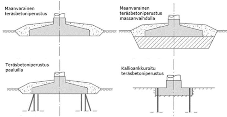
Kuva 3-2. Tuulivoimalaitosten perustamistekniikoita.
