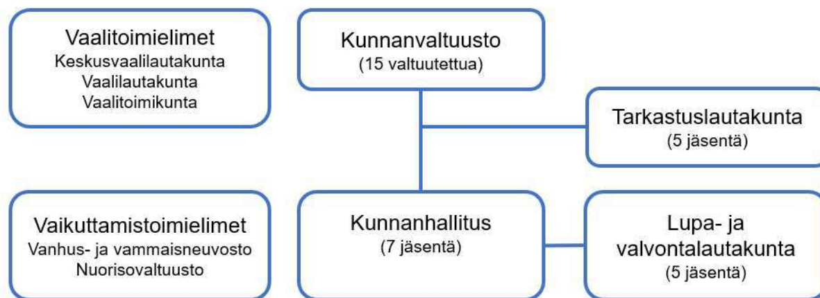
Kuva 2. Toimielinorganisaatio.
