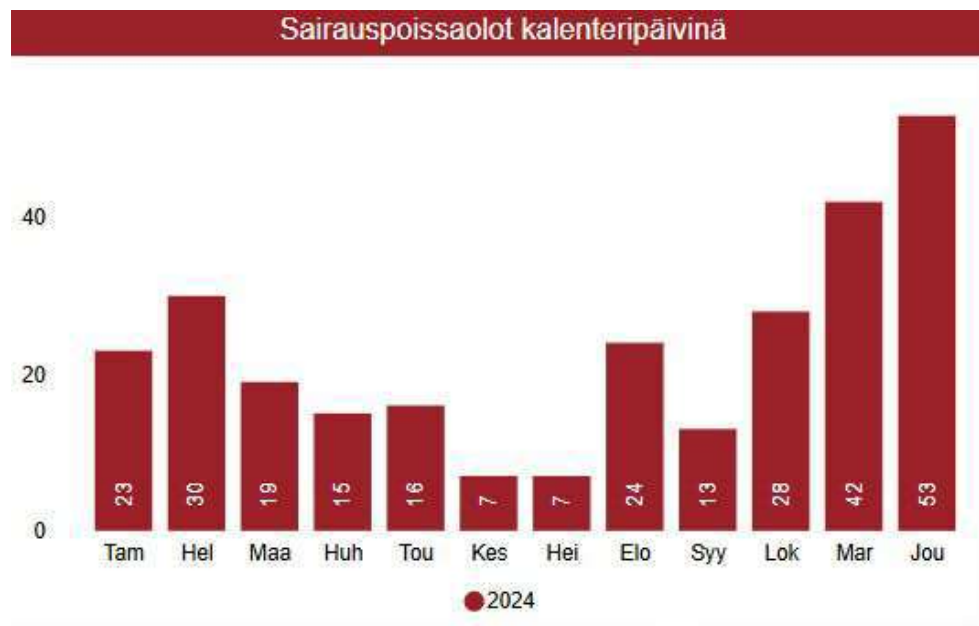
Kuva 11. Sairauspoissaolot kalenteripäivinä.
