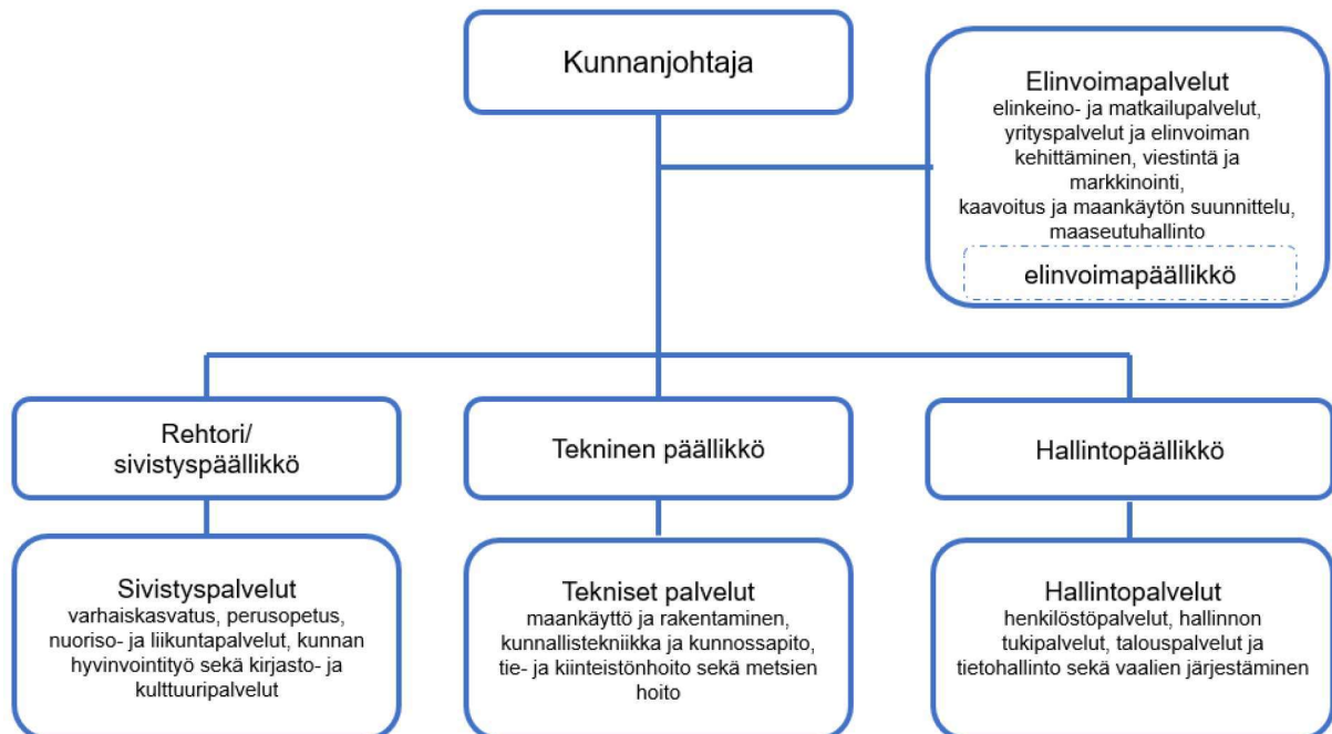
Kuva 1. Henkilöstöorganisaatio.
