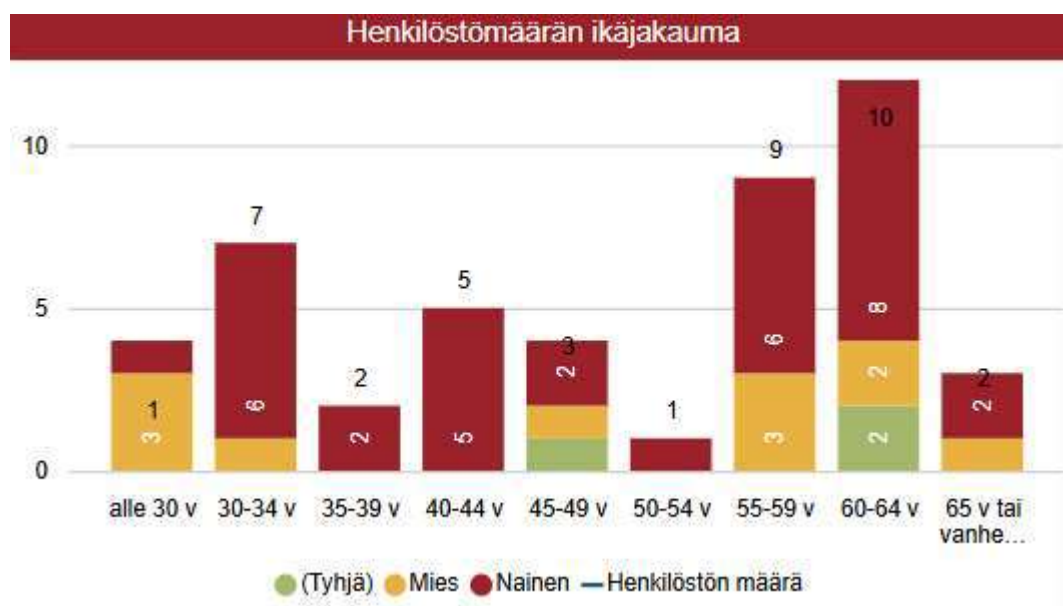
Kuva 9. Henkilöstön ikäjakauma.
